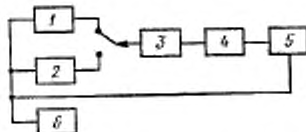
1—генератор, работающий в режиме «ВНЕШНЯЯ ЧМ»; 2—поверяемый генератор; 3—измеритель модуляции; 4—селективный вольтметр; 5—фазометр; 6—генератор модулирующего напряжения.
